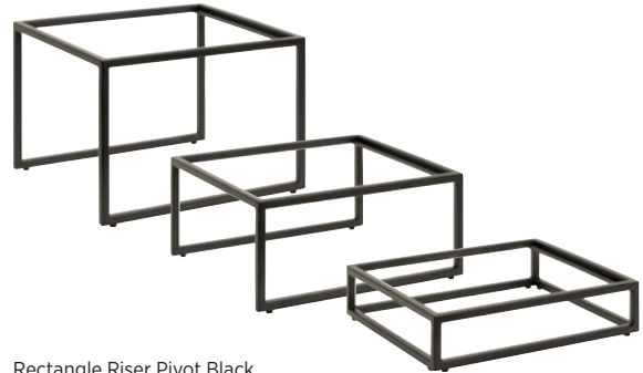
Rectangle Riser Pivot Black 7363MW338 L 11 1/2" W 13 7/8" H 9" CP 1 7363MW337 L 11 1/2" W 13 7/8" H 6" CP 1 7363MW336 L 11 1/2" W 13 7/8" H 3" CP 1
